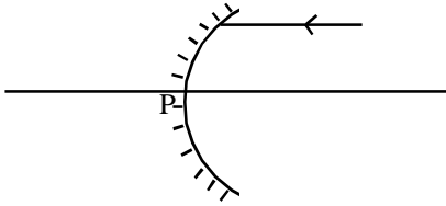
పుటాకార దర్పణం
