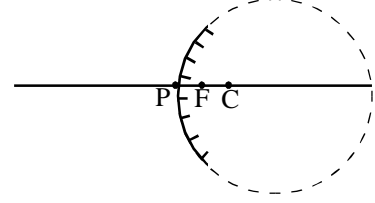
కుంభాకార దర్పణం
