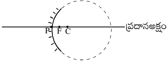
పుటాకార దర్పణం
