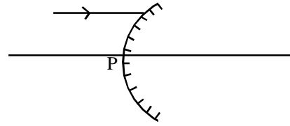
కుంభాకార దర్పణం
